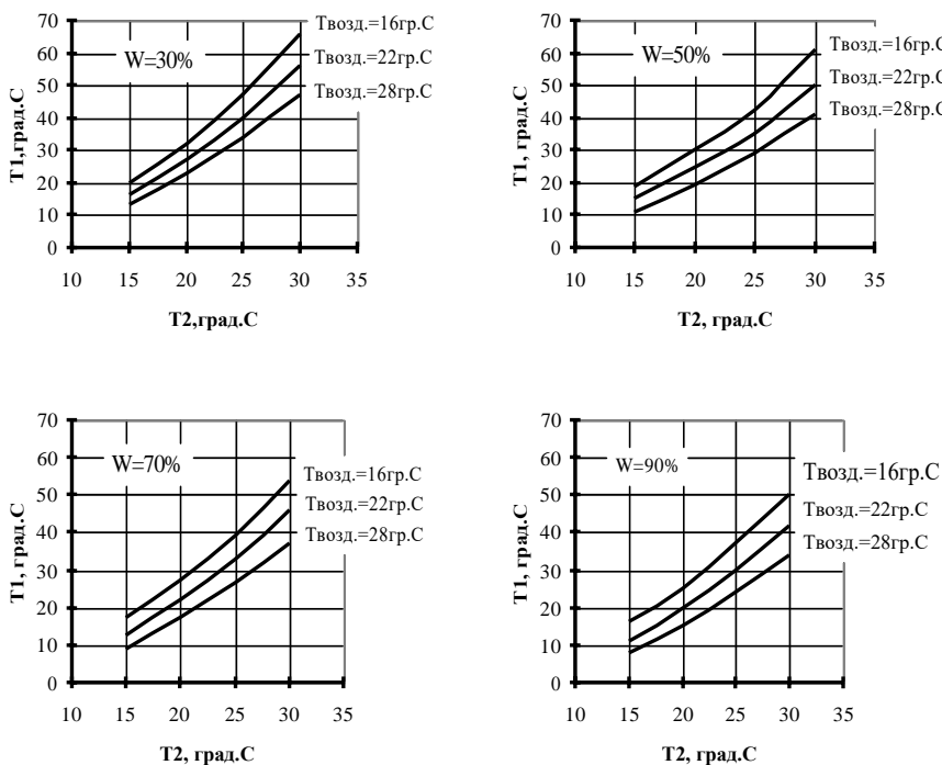
Рис.6. Графики охлаждения при расходе воды 30 \text{ м}^3/\text{ч} :
