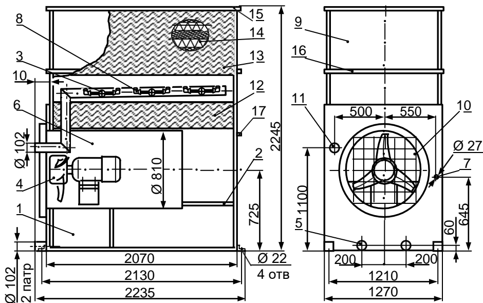
Рис. 1. Схема градирни
