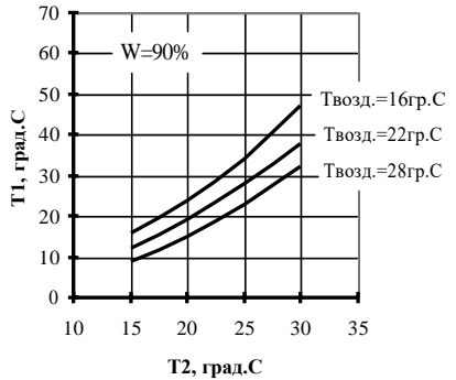
Рис.7. Графики охлаждения при расходе воды 40 \text{ м}^3/\text{ч} :
