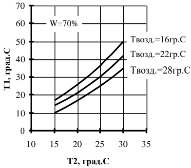
Рис.7. Графики охлаждения при расходе воды 40 \text{ м}^3/\text{ч} :
