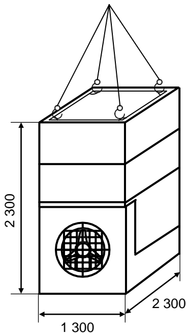
Рис. 5. Схема строповки градирни.
