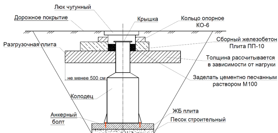
Схема монтажа подземного оборудования под проезжую часть
