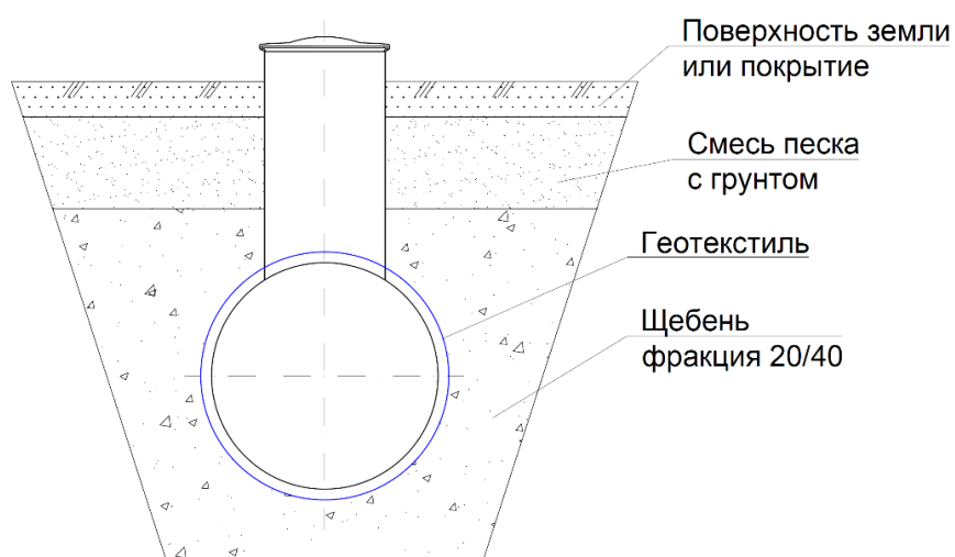
Схема монтажа дренажных тоннелей
